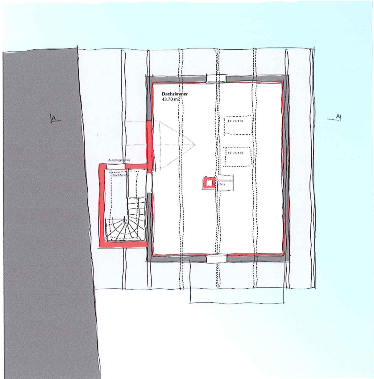
Dachgeschoss 1:100
