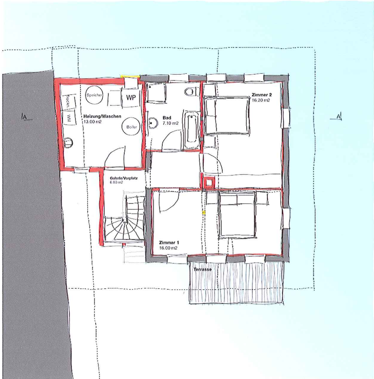
Obergeschoss 1:100
