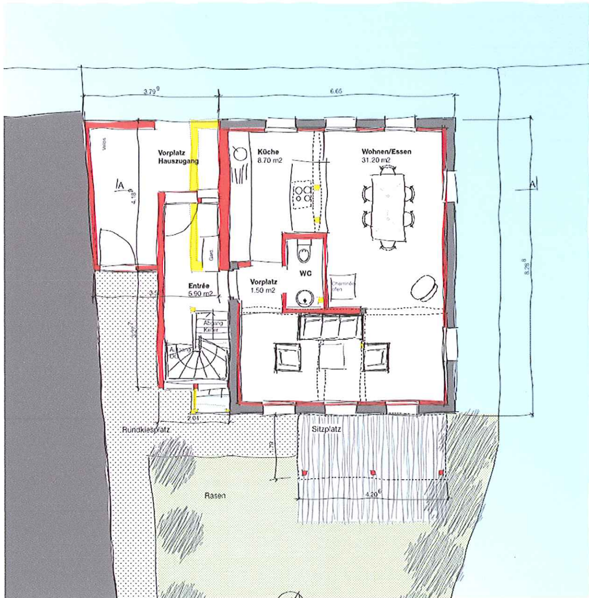
Erdgeschoss 1:100
