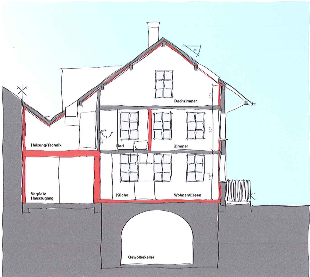
Schnitt 1:100
